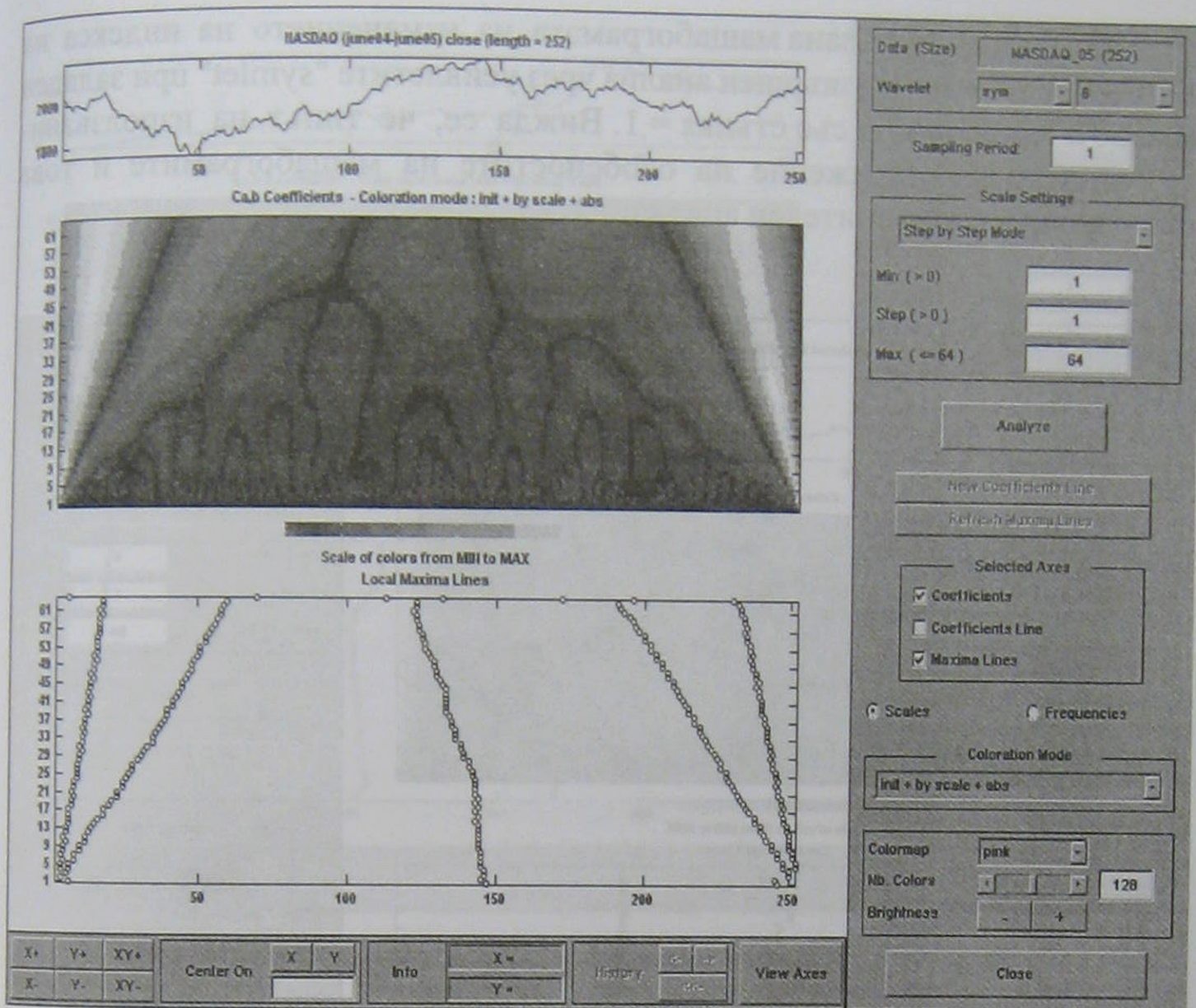
Фиг. 4 Анализ на NASDAQ чрез symlet wavelets за периода 7 юни 2004 - 6 юни 2005 г.
