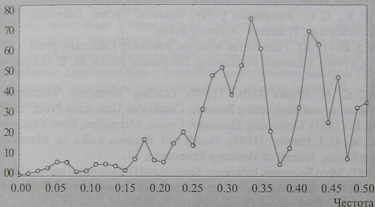
Фиг. 9. Крос-амплитуда за A_1/B_1
