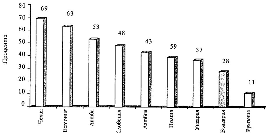
Фиг. 2. Относителен дял на предприятията, предлагащи обучение в страните, кандидатстващи за членство в ЕС
