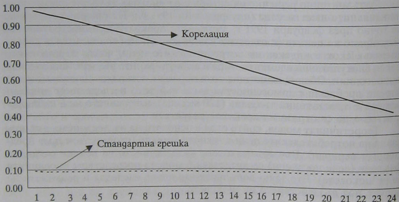
Фиг. 2. Автокорелационна функция на потребителските цени
