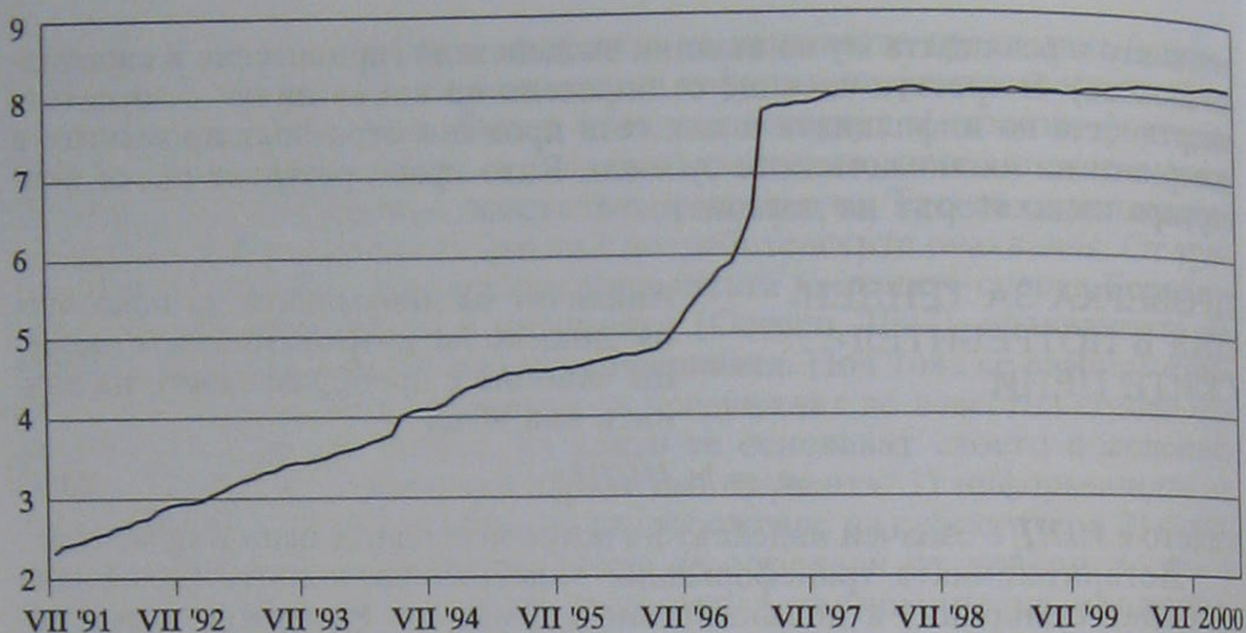
Фиг. 1. Динамика на потребителските цени (логаритми на базисните индекси)
