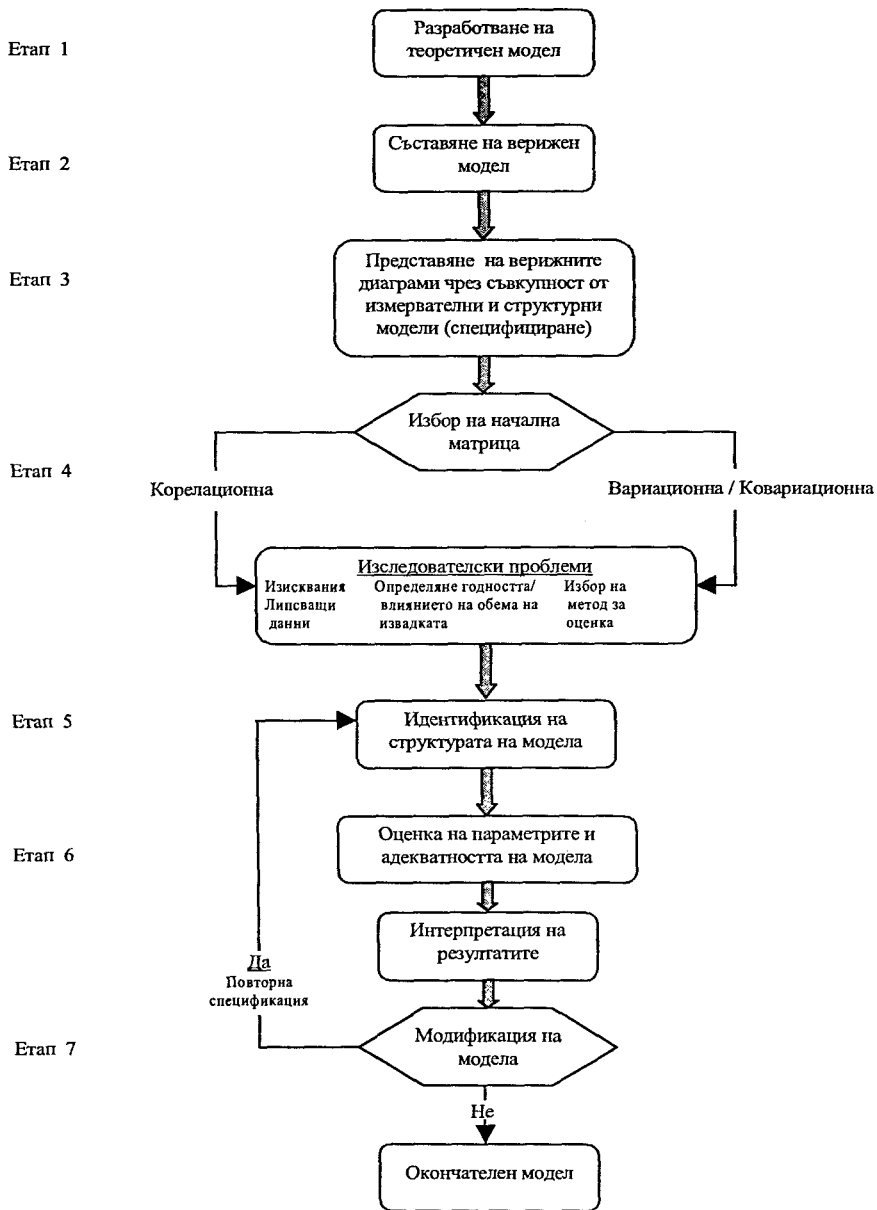
Фиг. 1. Етапи при извършването на латентно-структурен анализ
