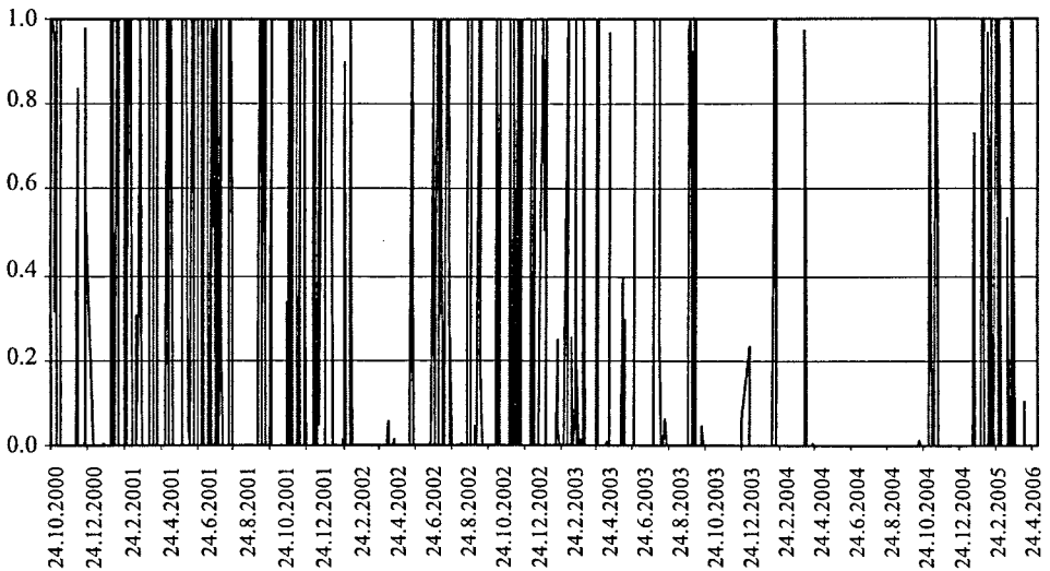
Фиг. 4. Функция на прехода във времето при LSTAR модела
