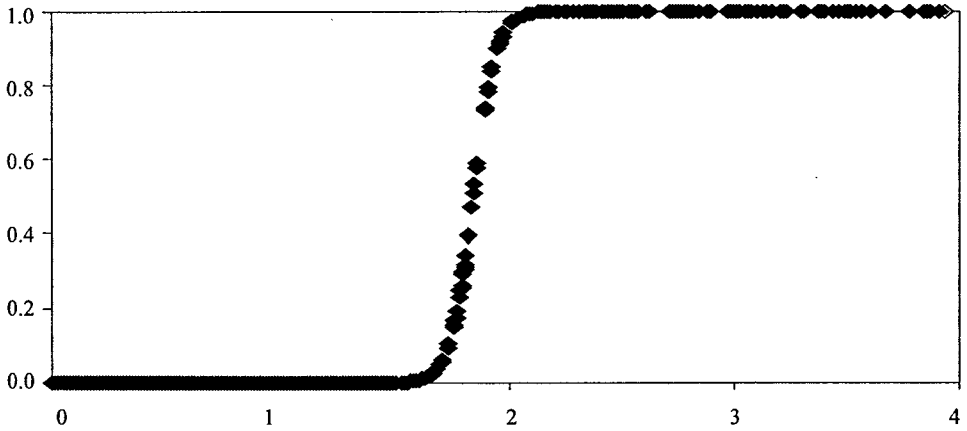
Фиг. 3. Функция на прехода в зависимост от променливата на прехода в LSTAR модела
