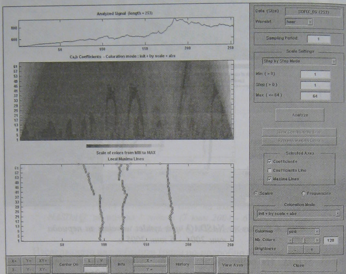
Фиг. 5. Анализ чрез уейвлети на Haar на изменението на индекса SOFIX - за периода 7 юни 2004 - 7 юни 2005 г.
