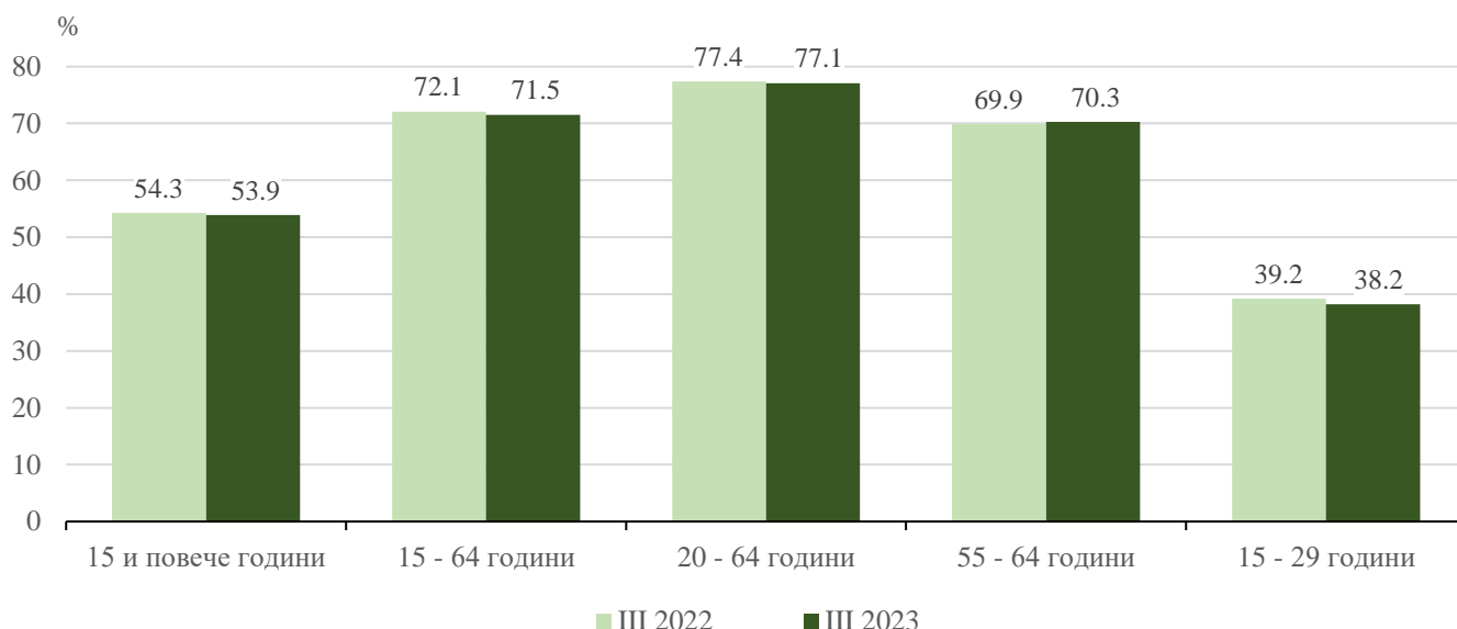
Фиг. 2. Коефициенти на заетост по възрастови групи през третото тримесечие на 2022 и 2023 година
