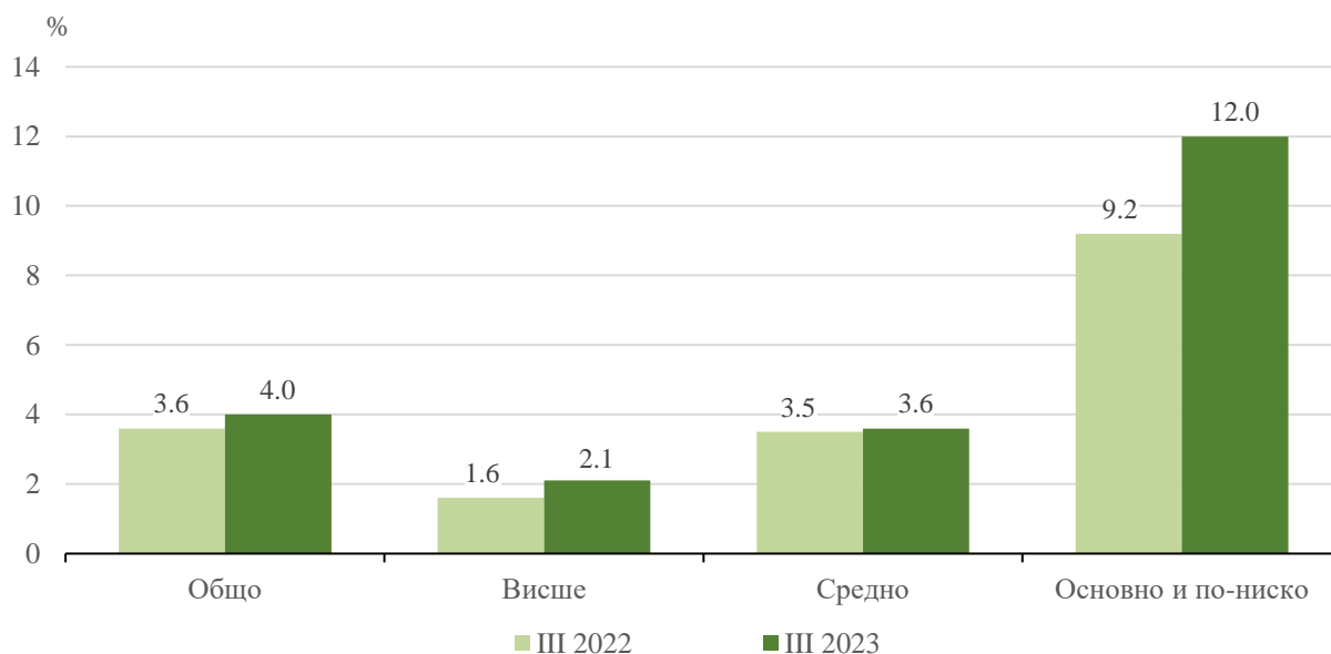
Фиг. 1. Коефициенти на безработица по степени на образование през третото тримесечие на 2022 и 2023 година
